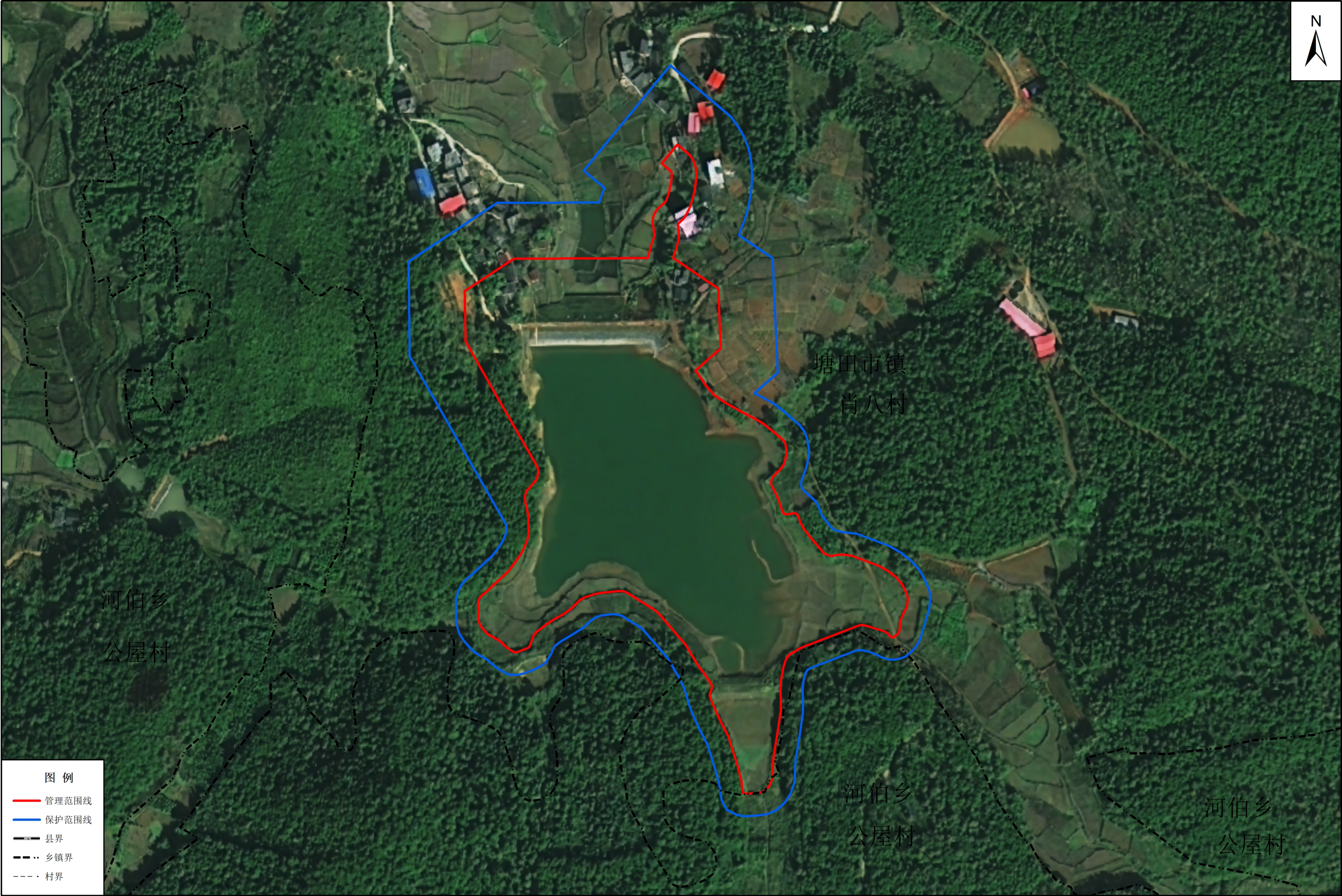
肖八水库管理与保护范围划界成果示意图
