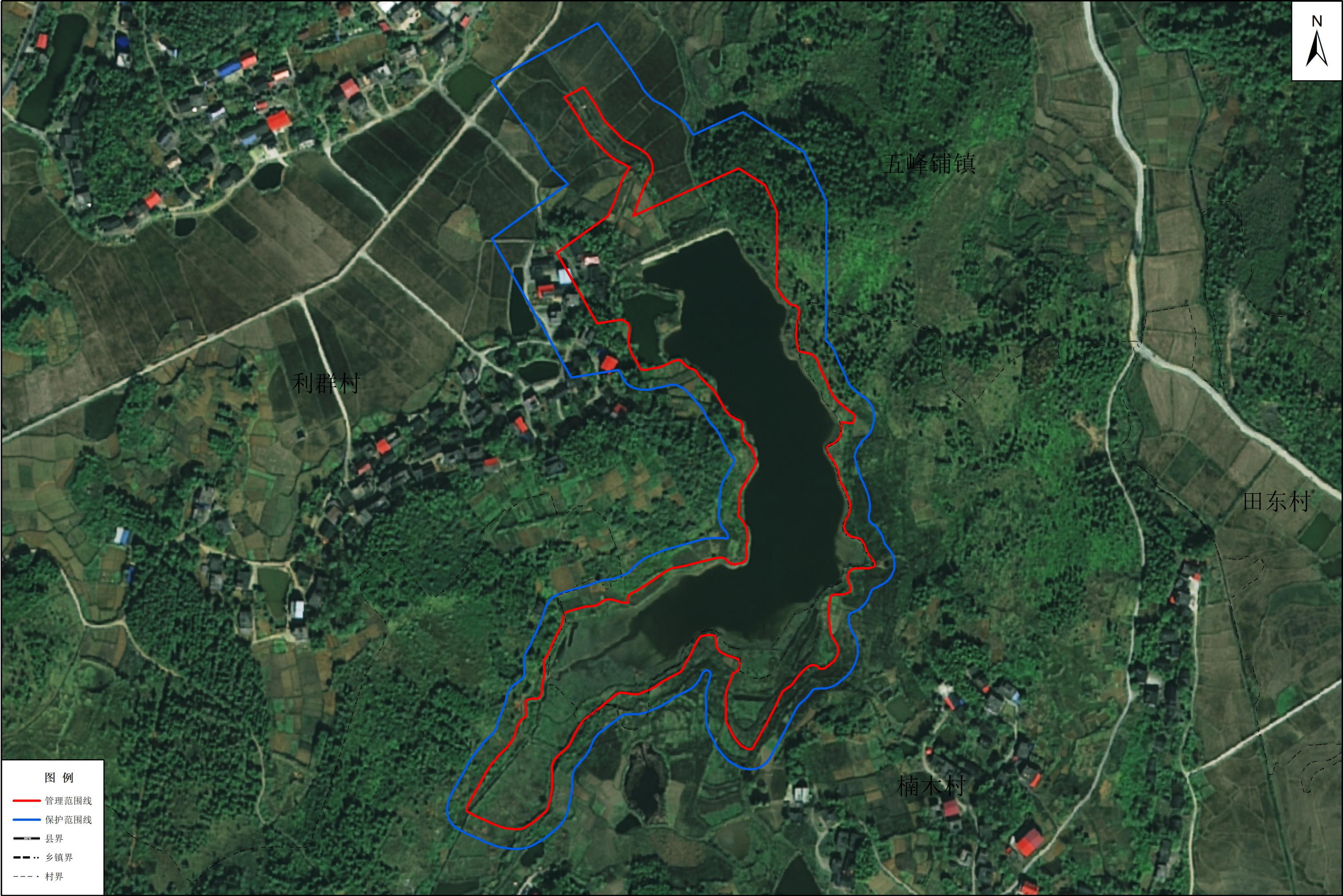
罗家冲水库管理与保护范围划界成果示意图
