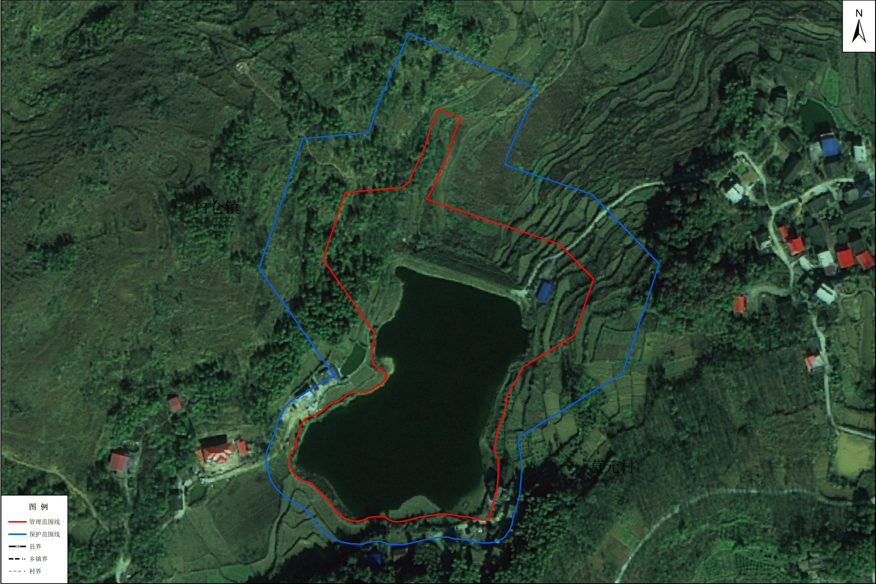
莲禾塘水库管理与保护范围划界成果示意图
