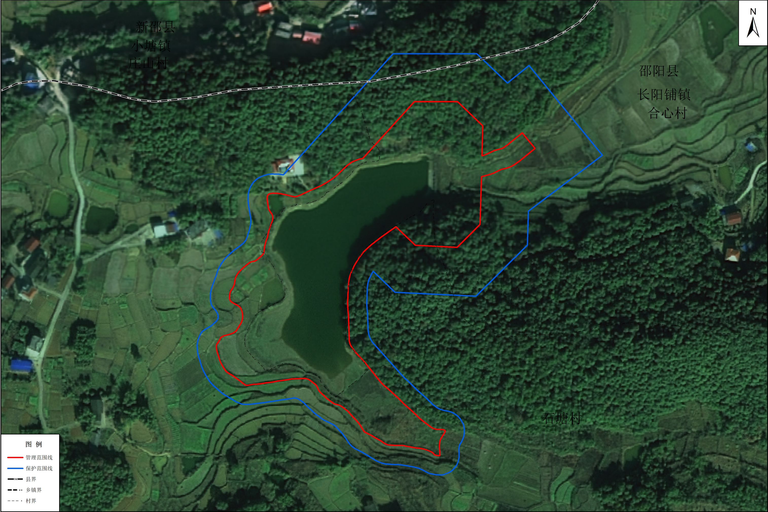
月致水库管理与保护范围划界成果示意图
